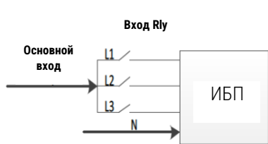
Схема входного реле для модели с одним входом
