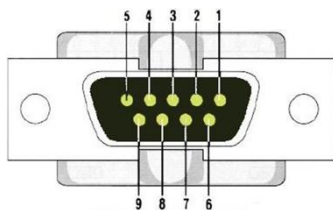
Порт DB9
