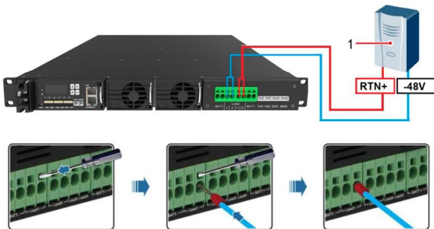
Рис. 4-9 Схема установки кабеля нагрузки
