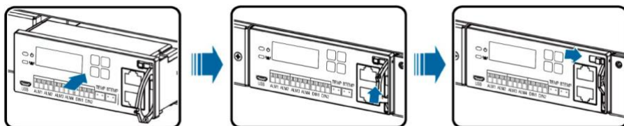
Рис. 7-4 Установка МА
