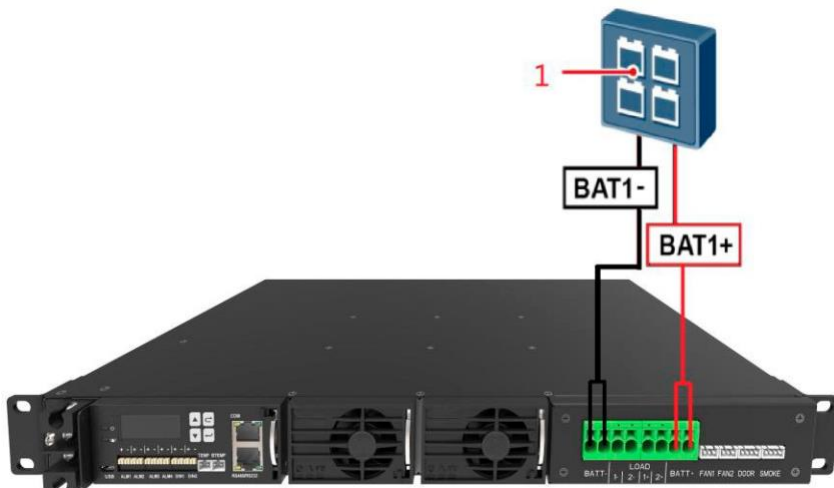
Рис. 4-10 Установка кабелей аккумуляторной батареи
