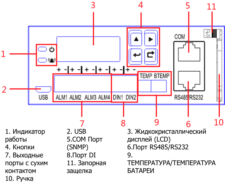
Рис. 3-1 Панель управления
