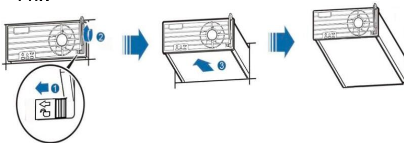
Рис. 7-1 Снятие выпрямителя
