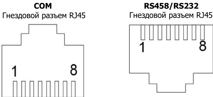
Рис.3-2 Контакты в порту COM и RS485/RS232
