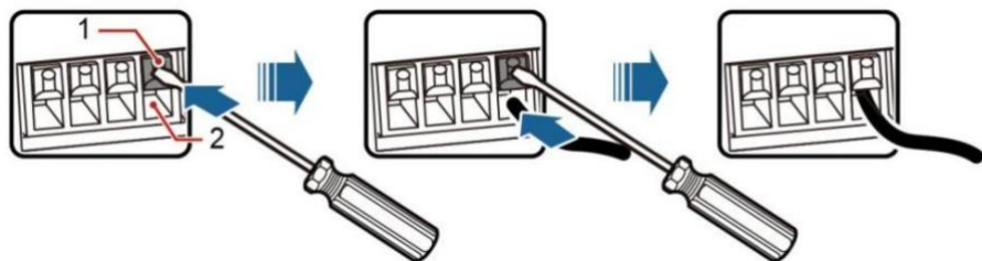
Рис. 4-4 Установка сигнального кабеля с сухим контактом
