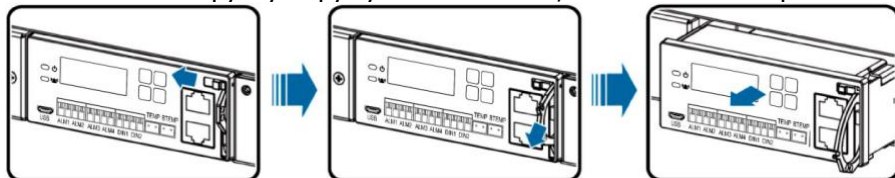
Рис. 7-3 Снятие МА
