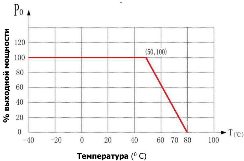
Рис. 2-2 Кривая зависимости выходной мощности от температуры окружающей среды
