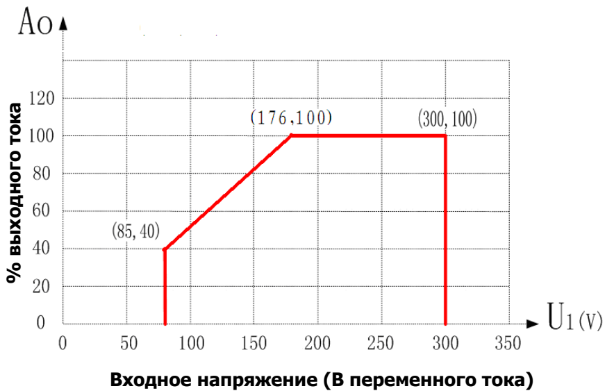
Рис. 2-3 Кривая выходная мощность-входное напряжение
