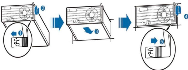
Рис. 7-2 Установка выпрямителя
