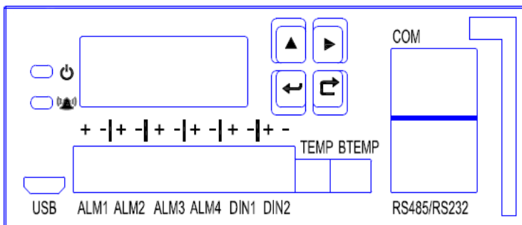
Рис. 4-3 Клемма с сухими контактами
