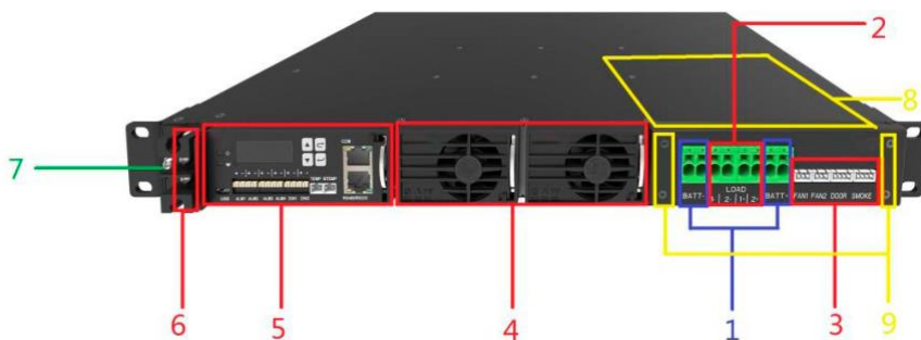
Рис. 1-1 Система питания постоянного тока ONTEK MRC 48-60
