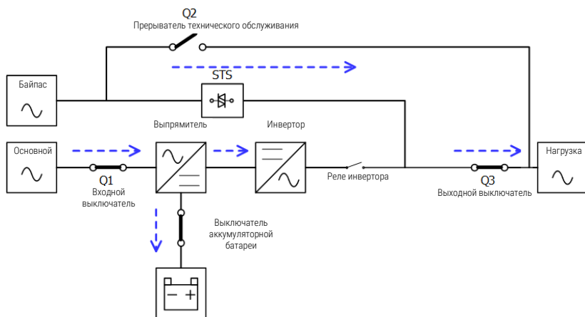
Рисунок 3-7 : Схема экономичного режима
