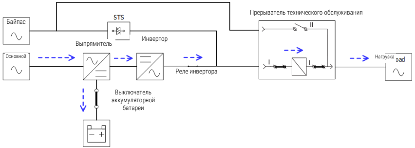
Рисунок 3-4 : Схема линейного режима
