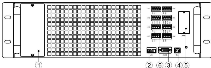
Рисунок 2-15. Модуль STS
