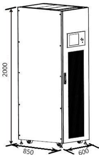
Рисунок 2-8 Размеры
