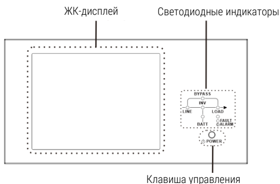
Рисунок 2-13. Панель управления
