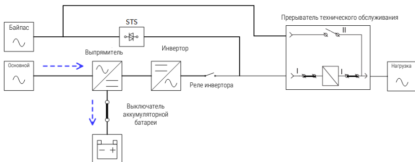
Рисунок 3-3 : Схема режима ожидания
