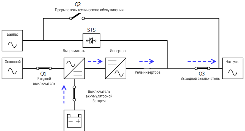
Рисунок 3-5: Схема линейного режима
