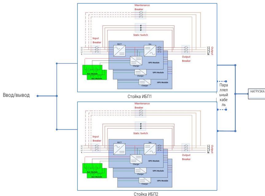
Рисунок 9-1 Подключение параллельной системы с тремя выключателями
