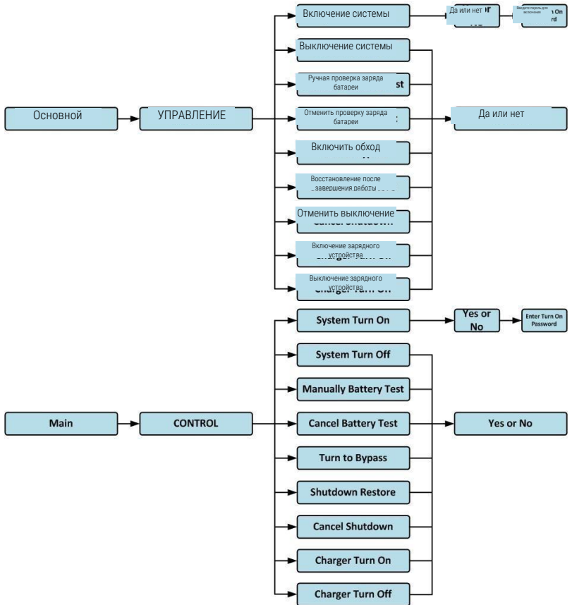
Рисунок 4-5. Дерево меню управления
