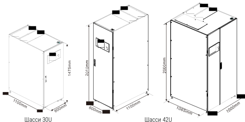
Рисунок 2-8 Размеры
