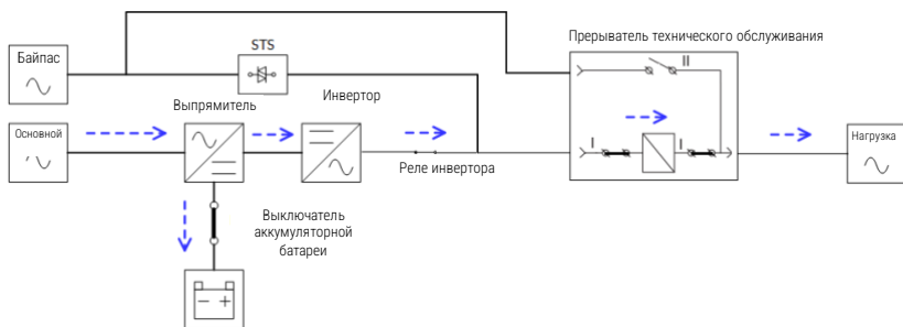
Рисунок 3-4: Схема линейного режима
