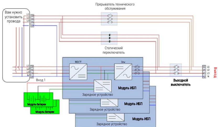
Электрическая схема для одного входа с двумя выключателями
