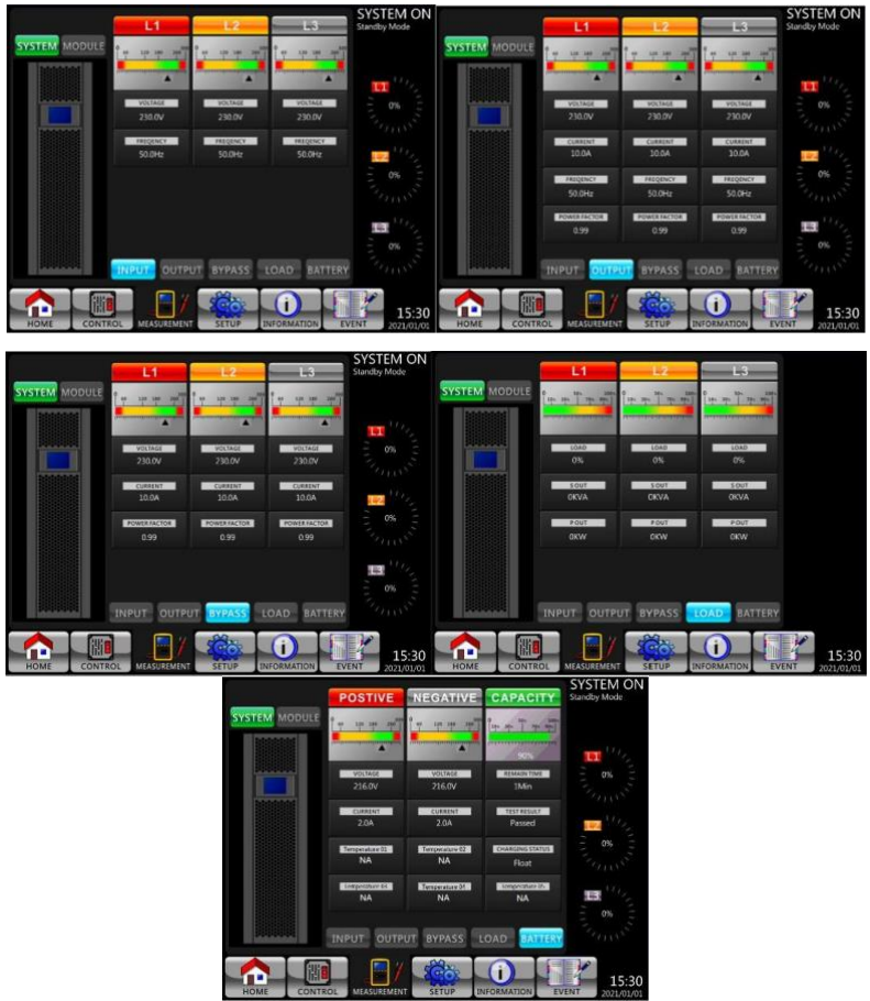
Рис. 4-9 Экраны системных измерений
