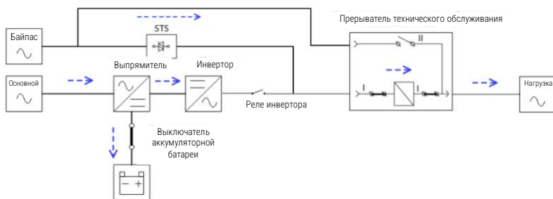
Рисунок 3-7: Схема экономичного режима
