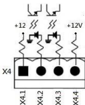
Рисунок 5-3 Порт состояния байпасного переключателя технического обслуживания
