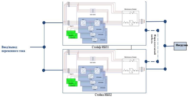
Рисунок 9-2 Подключение параллельной системы с одним байпасным выключателем технического обслуживания
