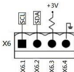
Рисунок 5-4 Порт определения температуры батарейного отсека
