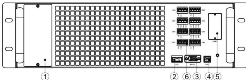
Рисунок 2-15. Модуль STS
