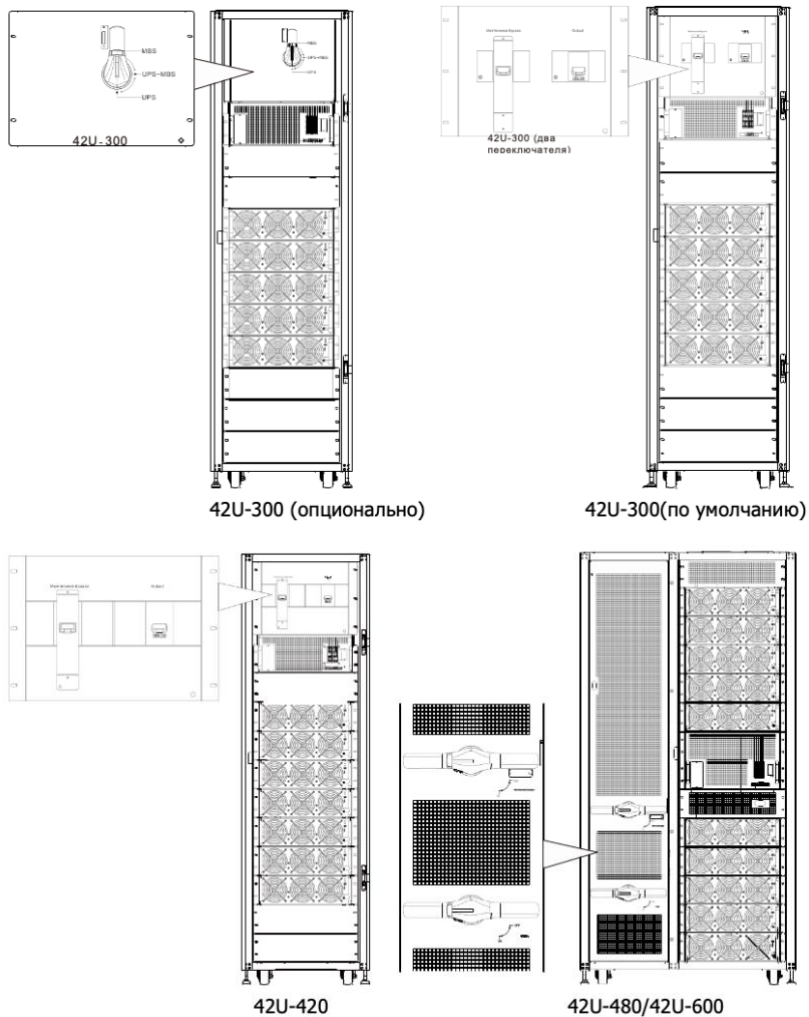
Рисунок 2-11. Переключатель (вид спереди)
