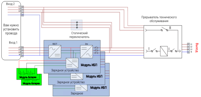
Схема подключения для двух входов с одним байпасным выключателем технического обслуживания
