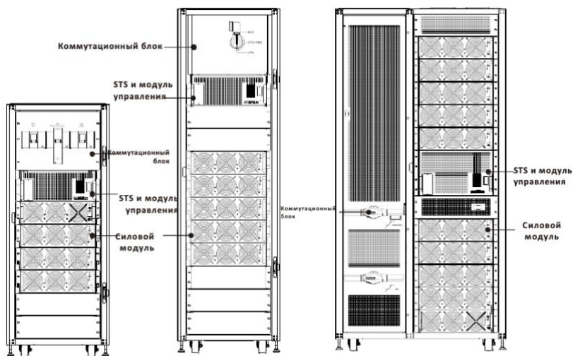
Рисунок 2-14. Вид спереди
