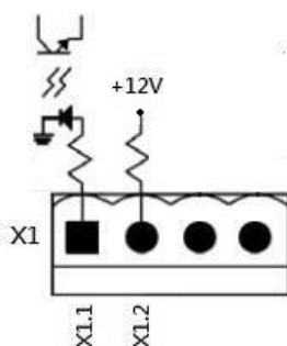
Рисунок 5-2 Удаленный входной порт EPO
