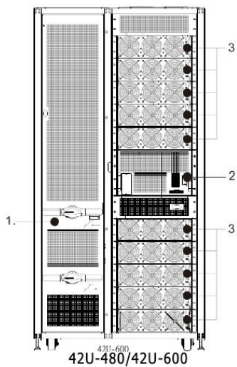
Рисунок 2-9 Вид спереди
