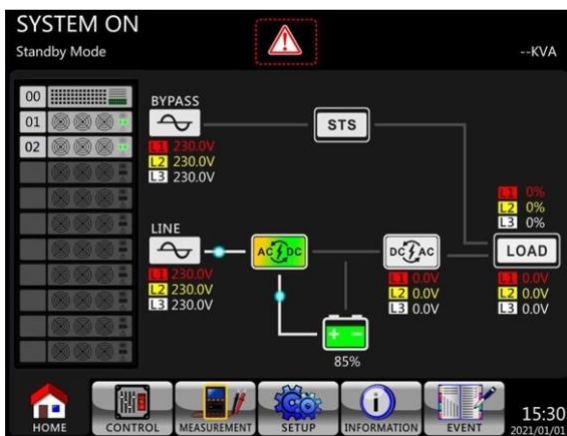
Рисунок 4-25 Экран предупреждения о тревоге
