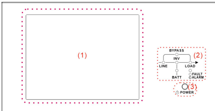
Рисунок 4-1 Панель управления
