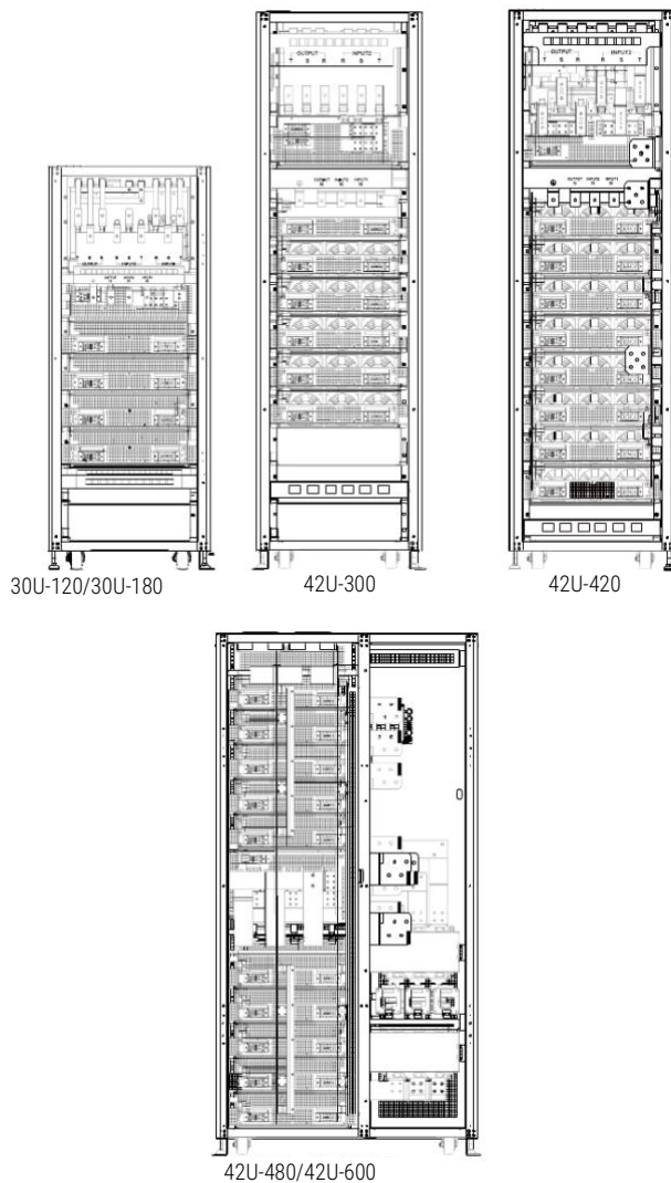
Рисунок 2-10 Вид сзади
