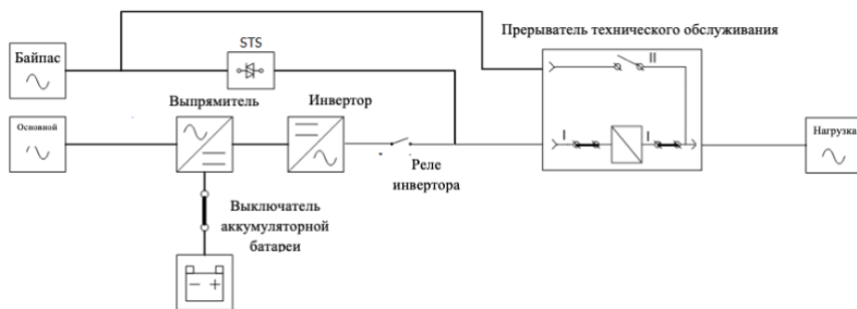
Рисунок 3-8: Схема режима выключения
