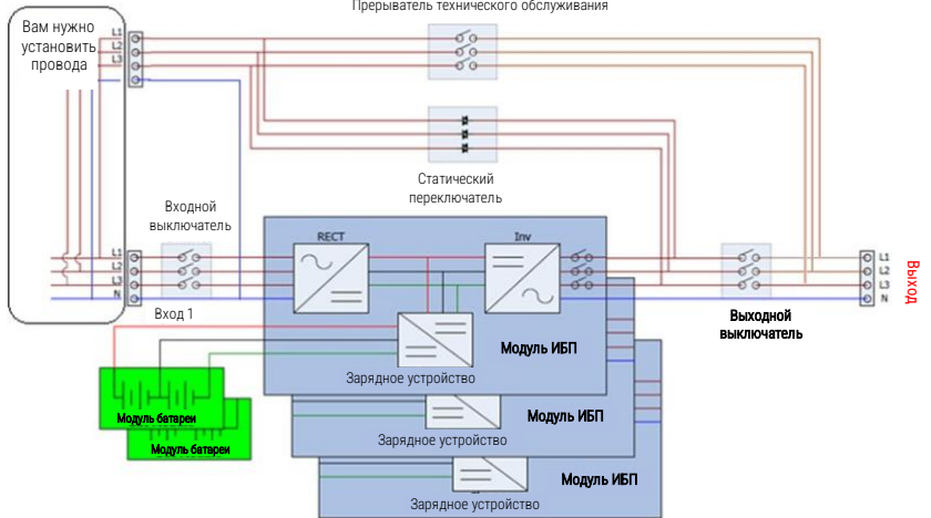
Схема подключения для одного входа с тремя выключателями
