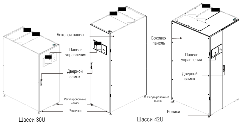
Рисунок 2-7 Внешний вид
