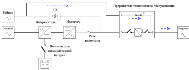
Рисунок 3-9: Схема режима обхода технического обслуживания
