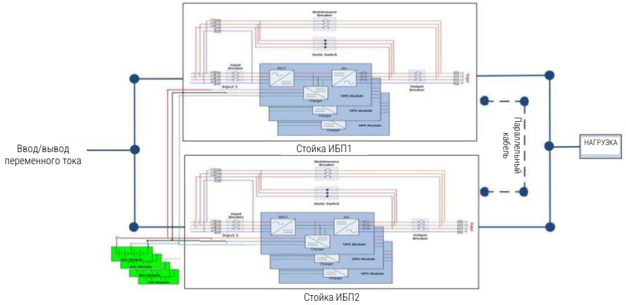
Рисунок 9-1 Подключение параллельной системы с тремя выключателями
