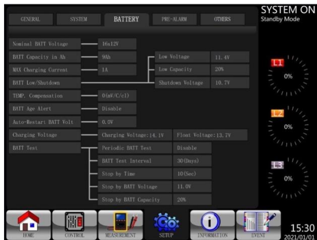
Рис. 4-17 Экран «Настройка-аккумулятор»
