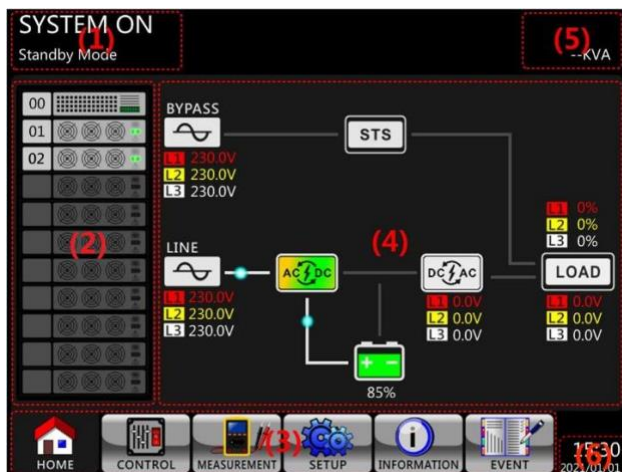
Рисунок 4-3. Главный экран
