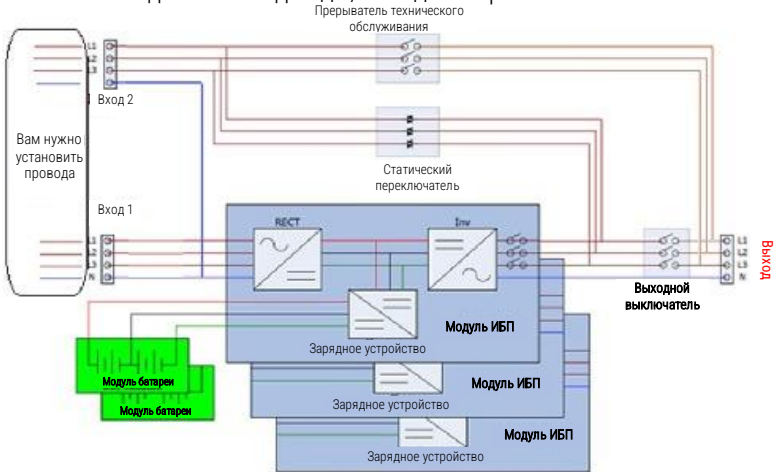
Электрическая схема для двух входов с двумя переключателями
