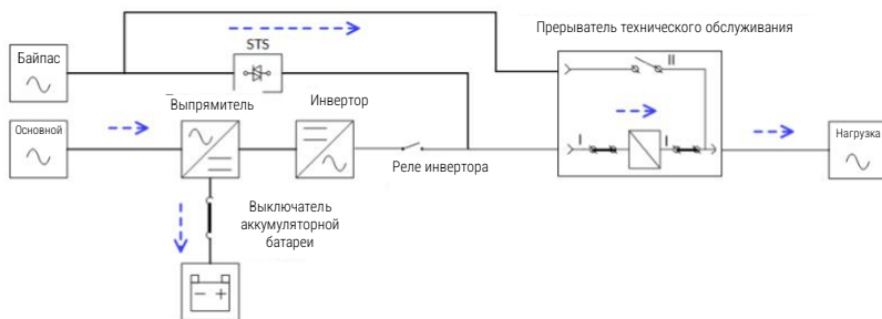
Рисунок 3-6: Схема режима байпаса
