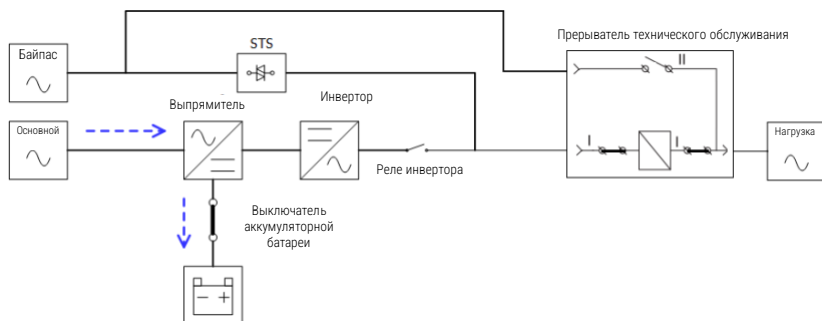
Рисунок 3-3: Схема режима ожидания
