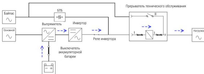
Рисунок 3-5: Схема линейного режима
