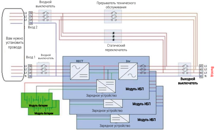
Схема подключения для двух входов с тремя выключателями
