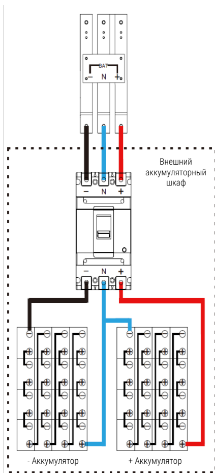
Рисунок 2-18. Подключение внешнего батарейного шкафа
