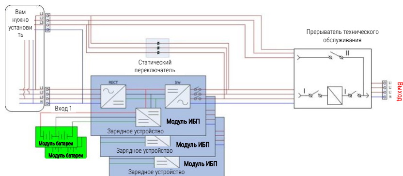
Схема подключения для одного входа с одним байпасным выключателем технического обслуживания
