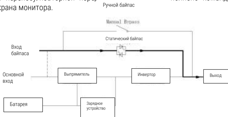
Рис. 1-4 Схема работы в режиме байпаса
